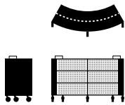
Shift+ Landscape con 2 módulos equipables por un lado, cada uno con 2 estantes with 2 modules which can be configured on both sides, each with 2 shelf inserts
